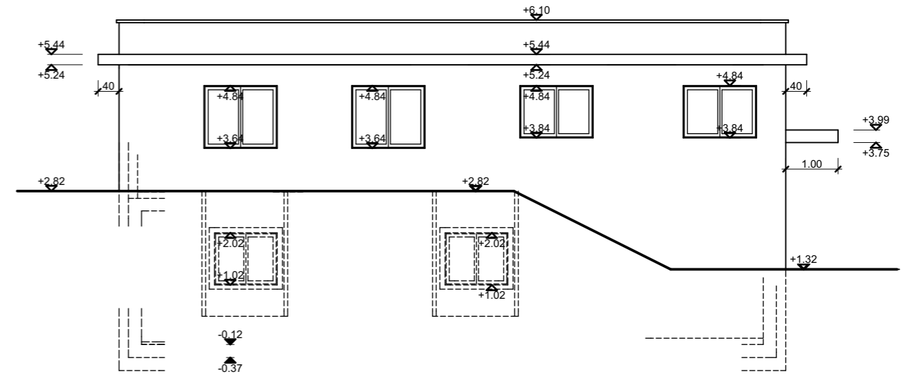
FACCIATA OVEST 1:100
