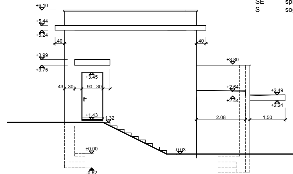
FACCIATA SUD 1:100
