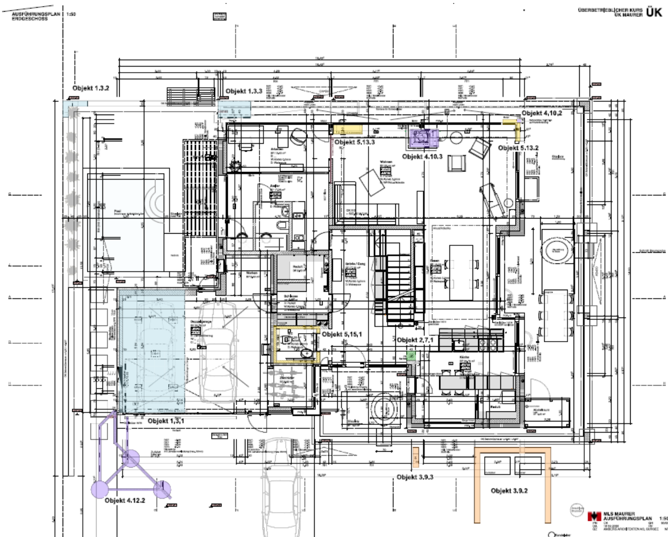
Abb. 2: Grundrissplan des Projektes
