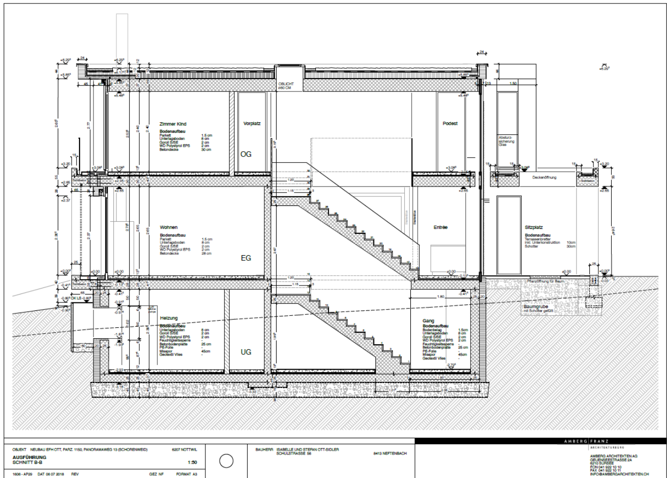
Abb. 3: Schnitt des Projektes
