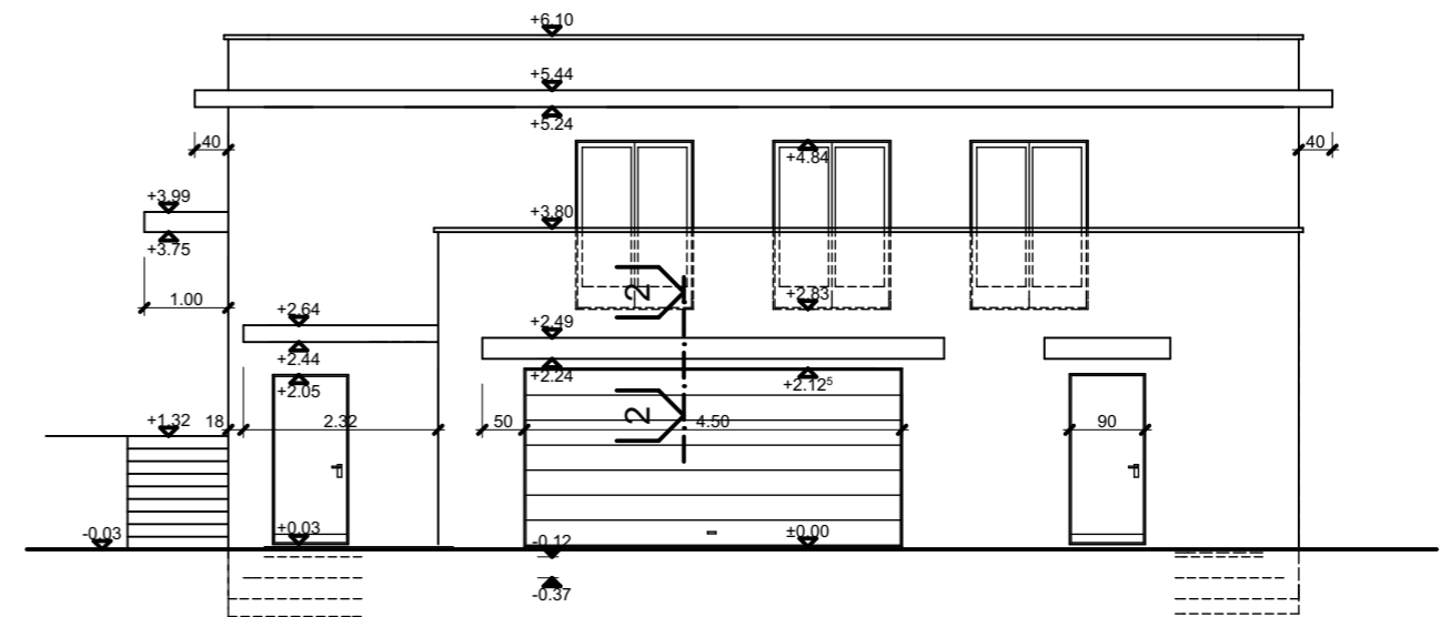
OSTFASSADE 1:100
