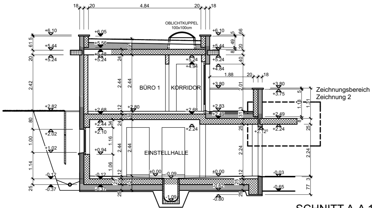
SCHNITT A-A 1:100
