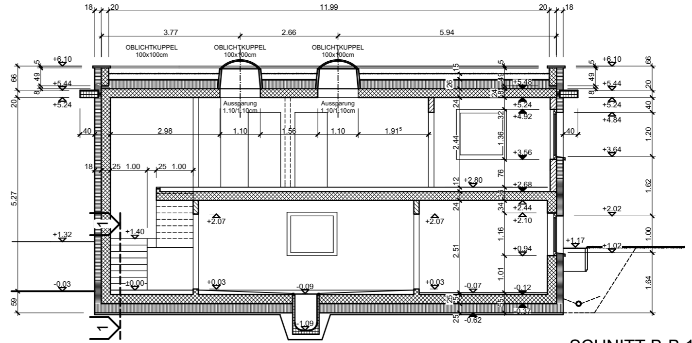
SCHNITT B-B 1:100
