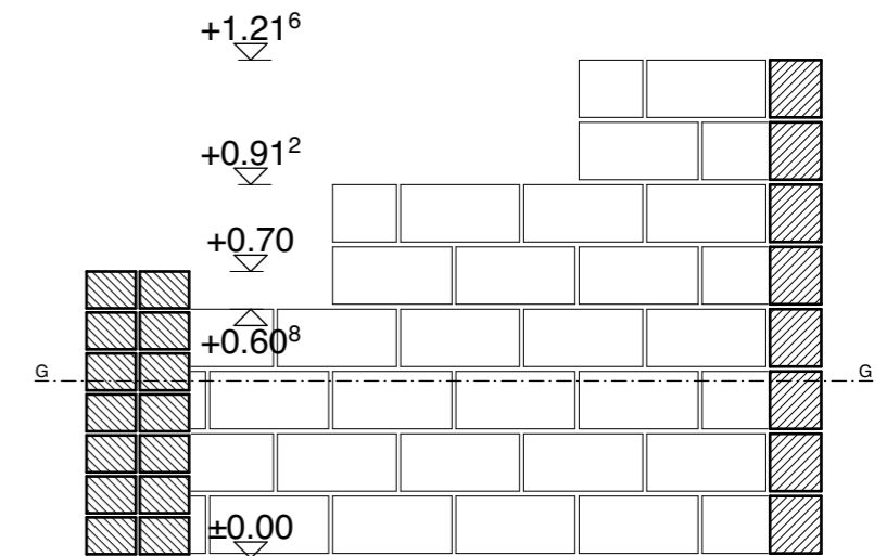
SCHNITT A-A (1:20)
